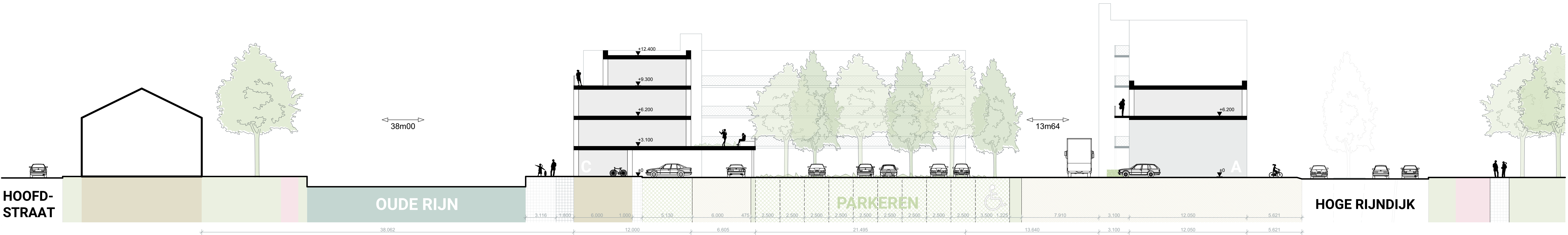
Doorsnede B-B
